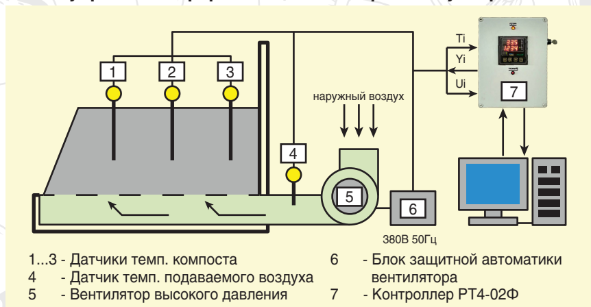
Фаза I. Ферментация компоста в открытом бункере
